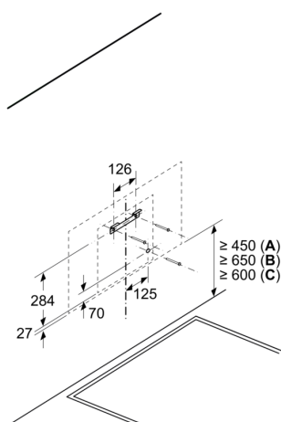
Mesures en mm Installation murale sans cheminée
