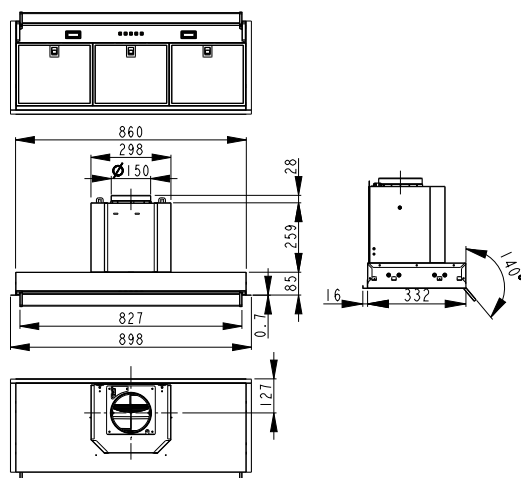
modèle 900 mm
