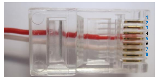
Figure : RJ-45 vue de dessous
