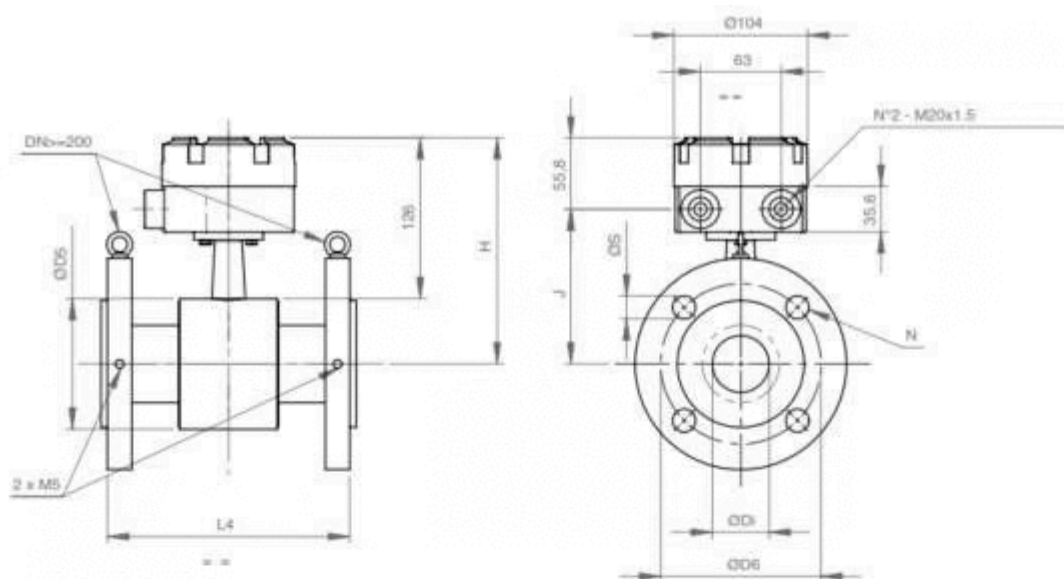
MUT2200EL PN 10 EN 1092-1
